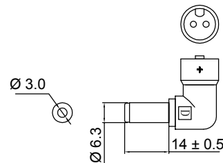
Adapterstecker 6 / Adapter plug 6 Typ „L“ / Type „L“ Material: PVC 20p, schwarz / Material: PVC 20p, black
