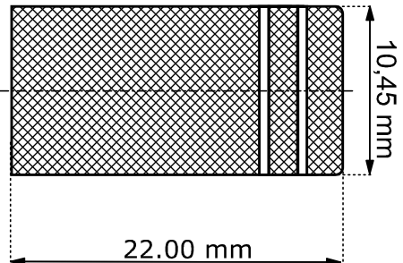
Gehäusehülse case sleeve
