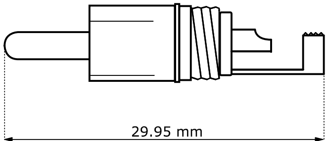
Kontaktträger contact mount
