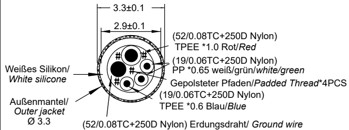
Diagramm Kabelquerschnitt Cross wire section diagram
